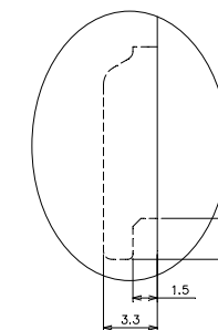
取付部A部詳細 (3/1)
