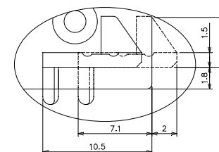
ロックレバー部(B部)詳細 (3/1)
