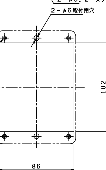
取付け穴加工参考図
