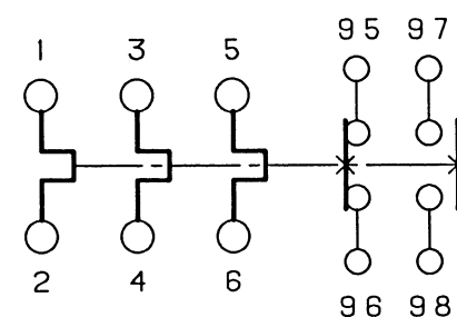
接点構成図
