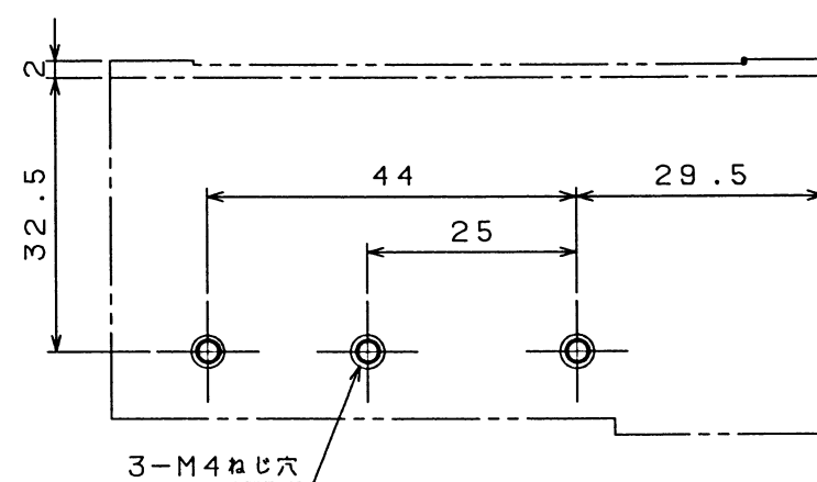
せん孔図
