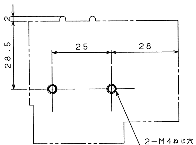
せん孔図
