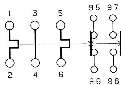
接点構成図
