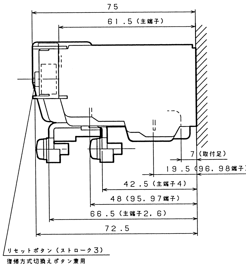
取付状態
