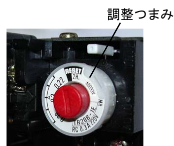
サーマルリレーの操作部
