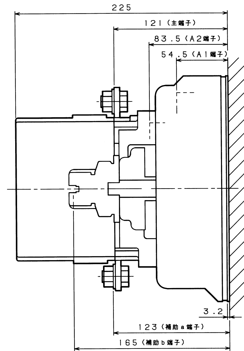
取付状態
