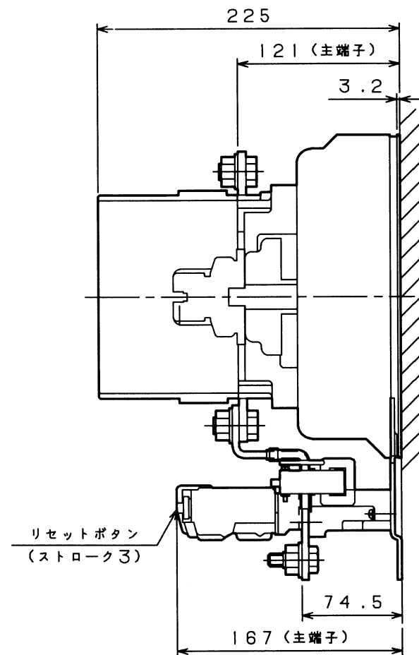
取付状態
