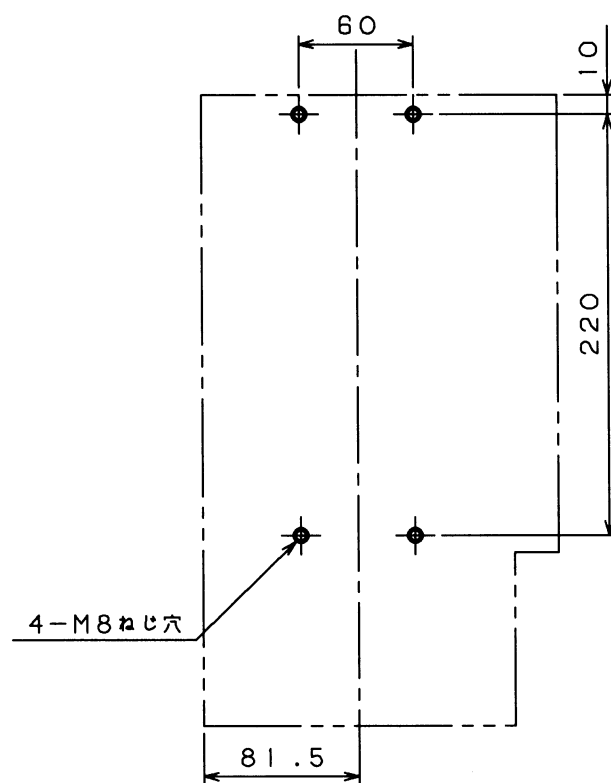
せん孔図
