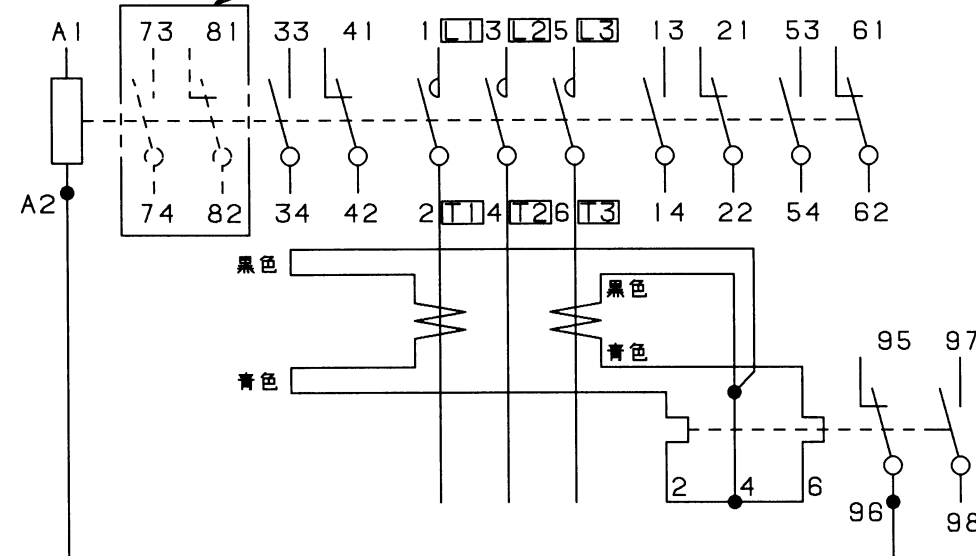
接点構成図
