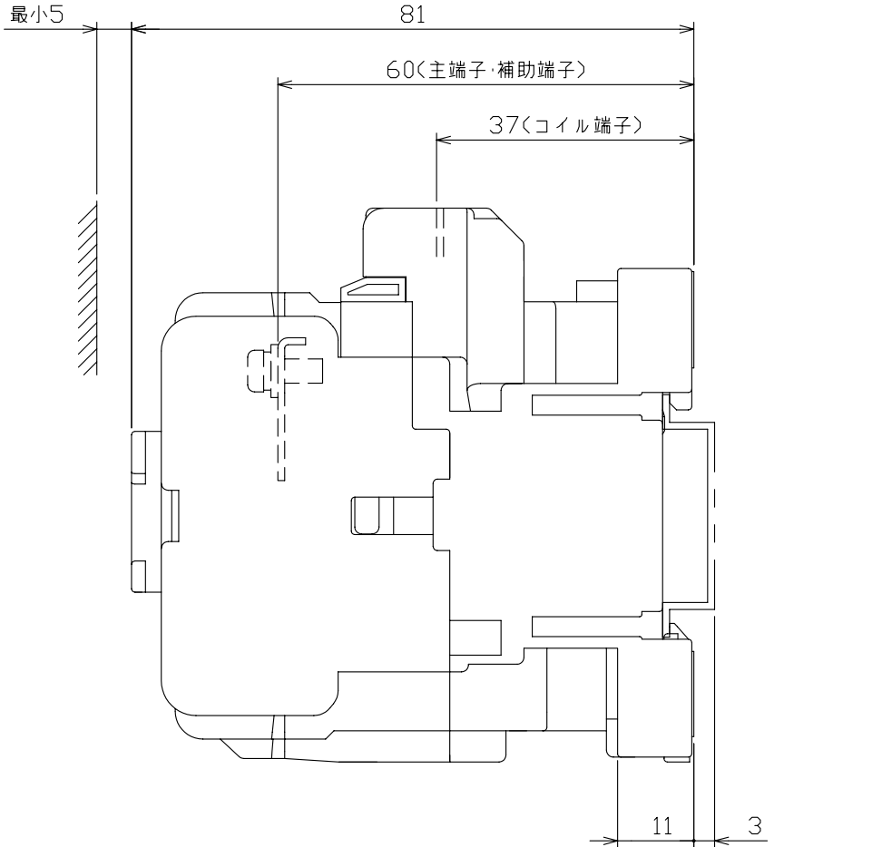
取付状態
