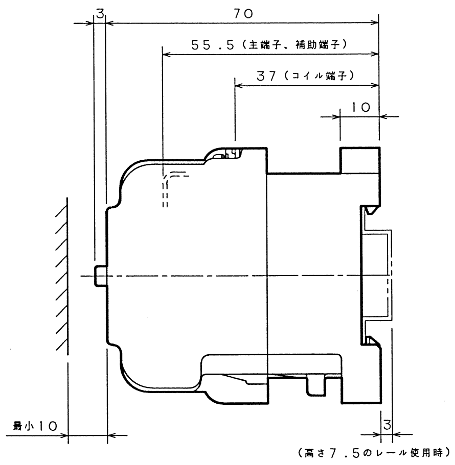
取付状態
