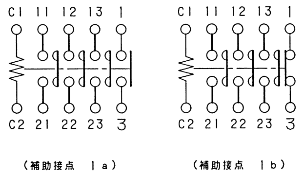
接点構成図
