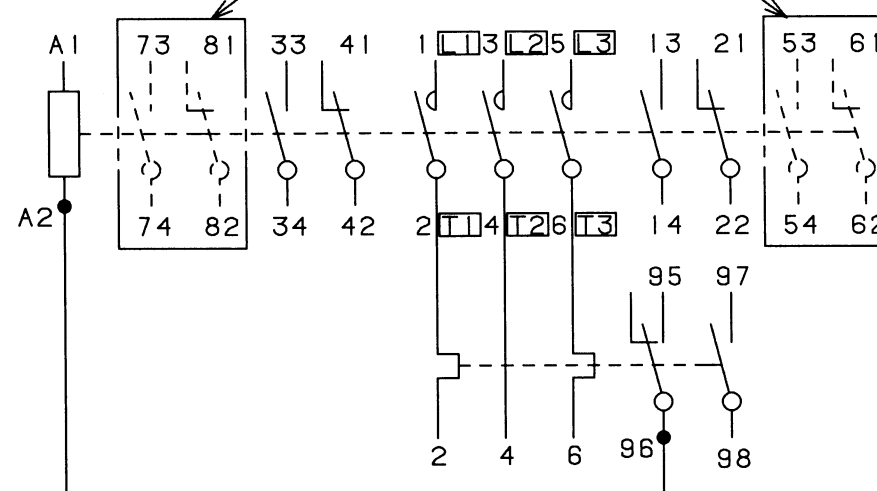
接点構成図
