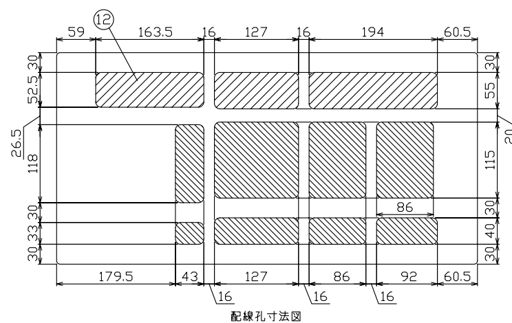
配線孔寸法図
