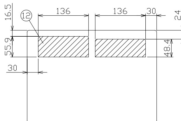
配線孔寸法図
