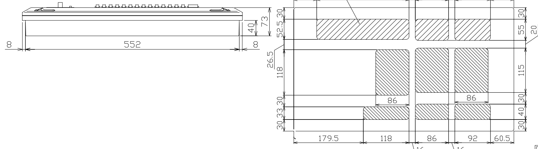
配線孔寸法図
