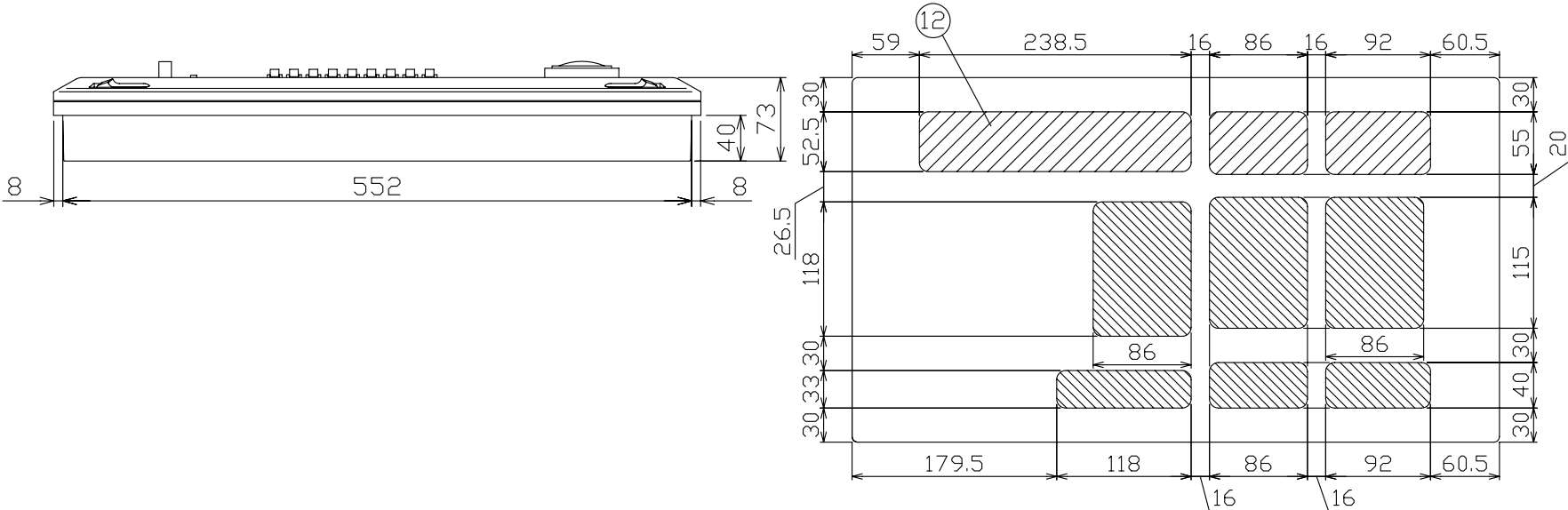
配線孔寸法図
