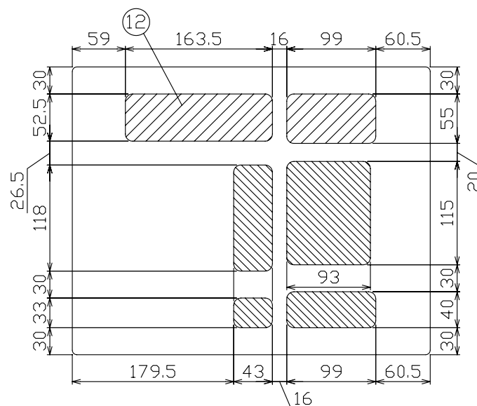
配線孔寸法図
