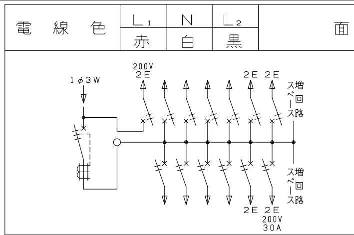
御 納 入 先 様 符号 部 分 品 名 備 考 1 キャビネット スチロール樹脂 UL-94 V-2 2 母線 銅板 60A容量(分岐30A容量) 3 主幹用漏電遮断器 50AF B,C, 5.0kA 30mA 高速形 4 配線用遮断器 30AF B,C, 2.5kA コード短絡保護機能付 5 充電部しゃへい板 ポリプロピレン樹脂 6 200V切替板 銅板 30A 容量 7 8 9 回路銘板 キャビネットカバー表面に貼付 10 100-200V切替説明書 キャビネットカバー裏面に貼付 11 配 線 孔 ノックアウト式 12 配 線 孔 //// 部開口, \\\\\ 部ノックアウト式 13 本体取付ネジ 4 - φ4.5 x 30 14 15 半埋込取付用サイドノック 4 - φ5 16 速結式アース中継端子 M 5 x 2 , 速結端子10P 17 18 電線(分岐部端子台～主幹) 600V HIV 電線 φ2mm 19 エコキュート用配線用遮断器 30AF B,C, 2.5kA コード短絡保護機能付
