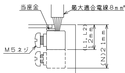
主幹用漏電遮断器端子構造
