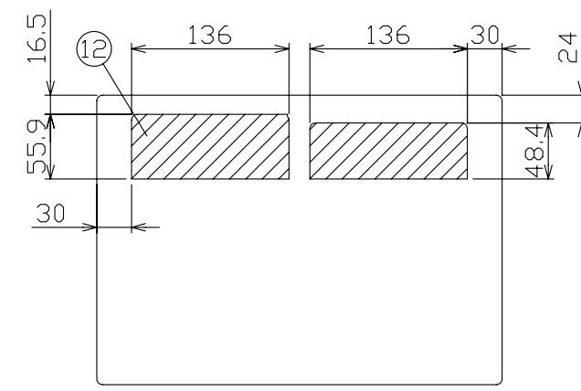
配線孔寸法図
