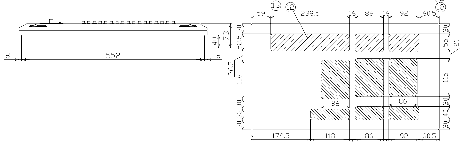
配線孔寸法図
