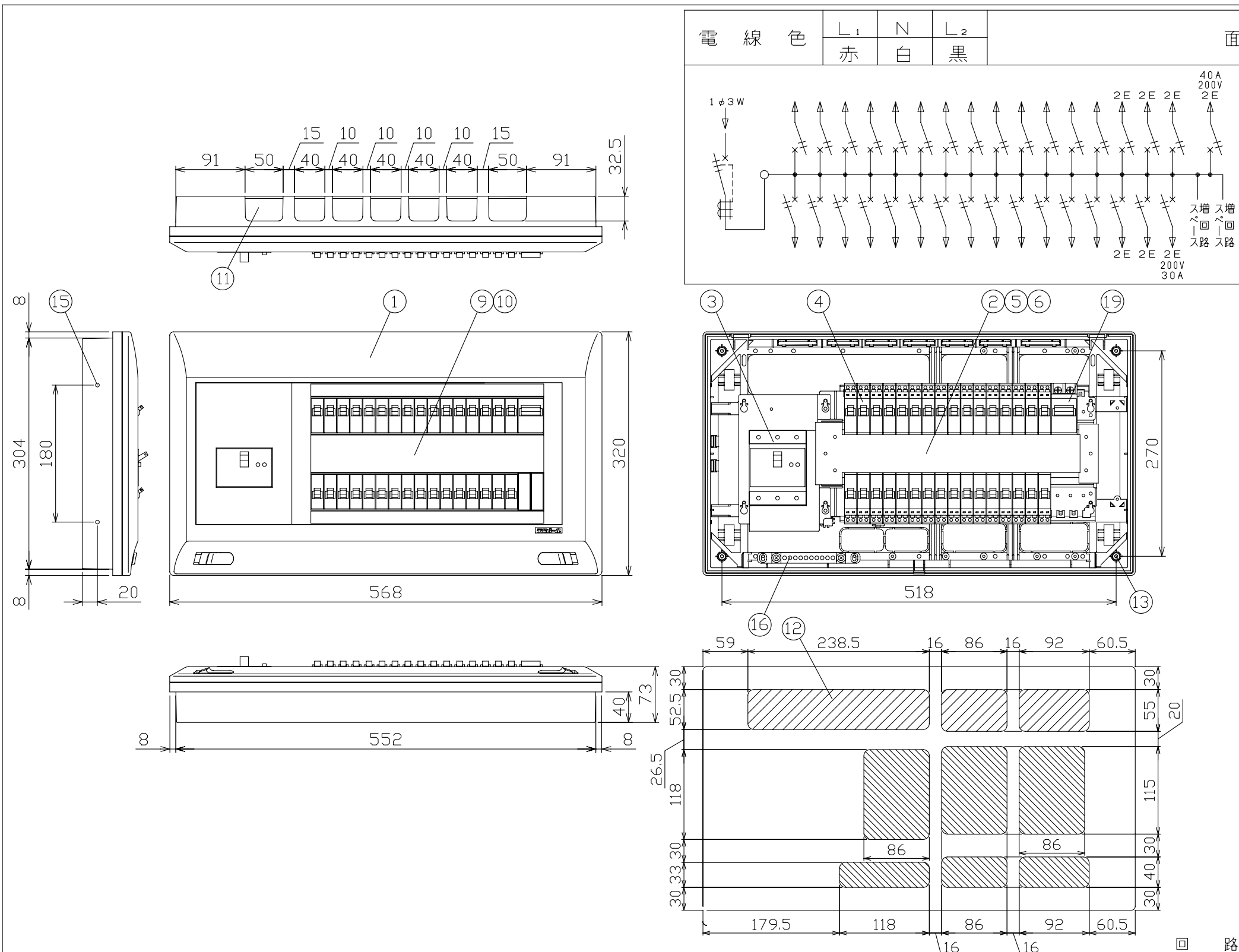
配線孔寸法図
