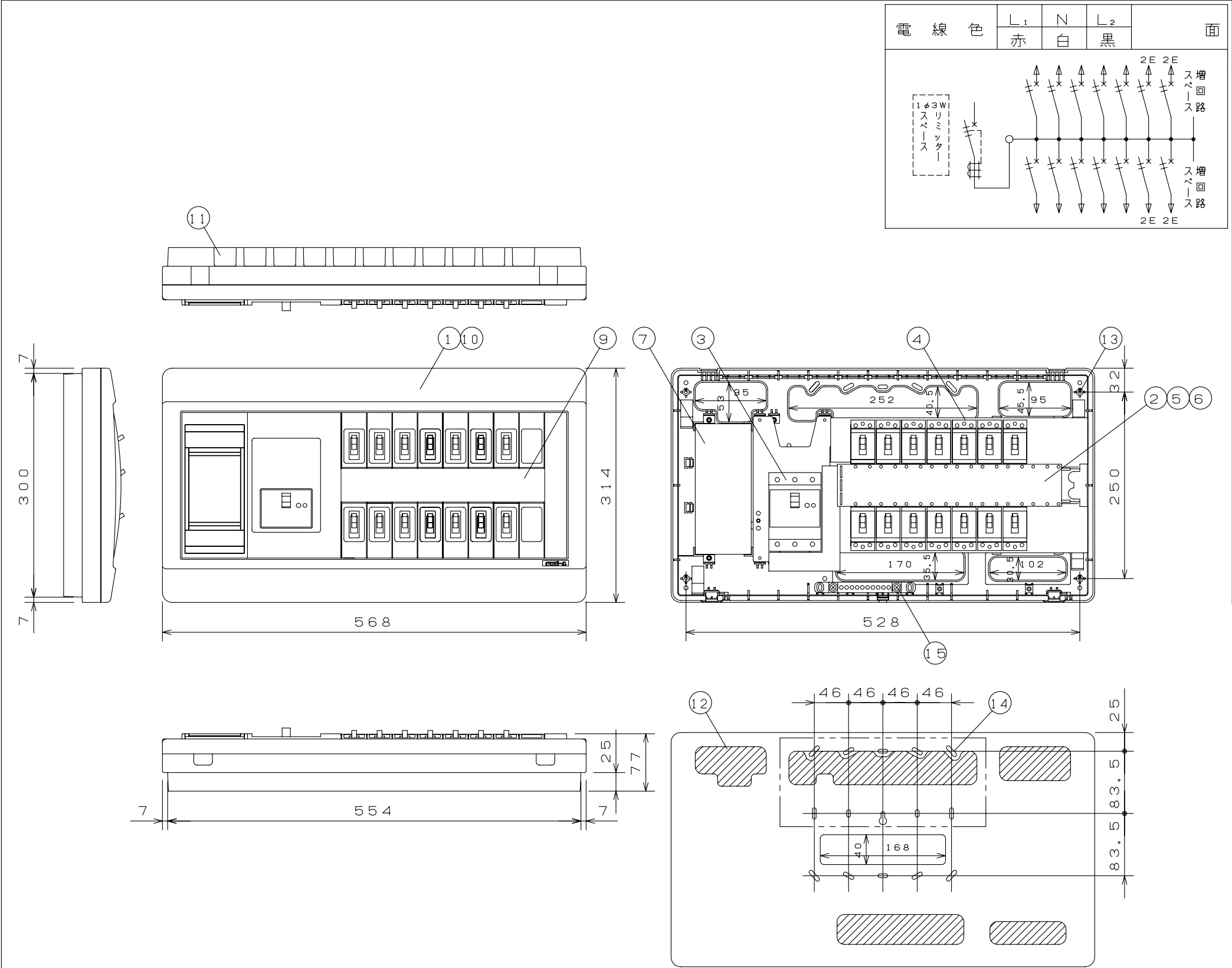
スイッチボックス位置図
