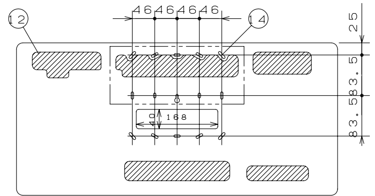
スイッチボックス位置図
