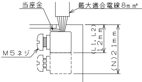
主幹用漏電遮断器端子構造
