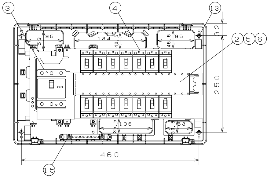
御納入先 様 符号 部 分 品 名 備 考 1 キャビネット スチロール樹脂 2 母線 銅板 100A容量(分岐30A容量) 3 主幹用漏電遮断器 75AF B,C, 5,0kA 30mA 高速形 4 配線用遮断器 30AF B,C, 2,5kA コード短絡保護機能付 5 充電部しゃへい板 ポリプロピレン樹脂 6 200V切替板 銅板 30A 容量 7 8 9 回路銘板 キャビネットカバー表面に貼付 10 100-200V切替説明書 キャビネットカバー裏面に貼付 11 配線用ロックアウト 9 - 30 x 25 12 配 線 孔 13 本体取付ネジ 4 - φ4 x 30 14 スイッチボックス取付穴 5個用スイッチボックス取付可能 15 速結式アース中継端子 M 5 x 2 , 速結端子10P 16 17 18 19
