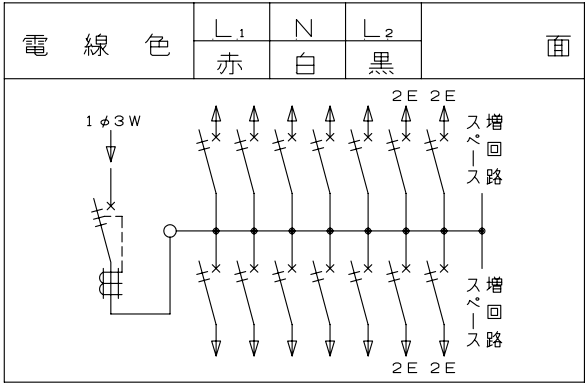
御納入先 様 符号 部 分 品 名 備 考 1 キャビネット スチロール樹脂 2 母線 銅板 100A容量(分岐30A容量) 3 主幹用漏電遮断器 75AF B,C, 5,0kA 30mA 高速形 4 配線用遮断器 30AF B,C, 2,5kA コード短絡保護機能付 5 充電部しゃへい板 ポリプロピレン樹脂 6 200V切替板 銅板 30A 容量 7 8 9 回路銘板 キャビネットカバー表面に貼付 10 100-200V切替説明書 キャビネットカバー裏面に貼付 11 配線用ロックアウト 9 - 30 x 25 12 配 線 孔 13 本体取付ネジ 4 - φ4 x 30 14 スイッチボックス取付穴 5個用スイッチボックス取付可能 15 速結式アース中継端子 M 5 x 2 , 速結端子10P 16 17 18 19
