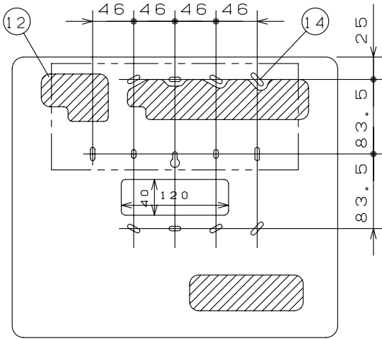
スイッチボックス位置図
