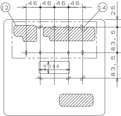
スイッチボックス位置図
