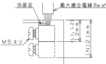
主幹用漏電遮断器端子構造
