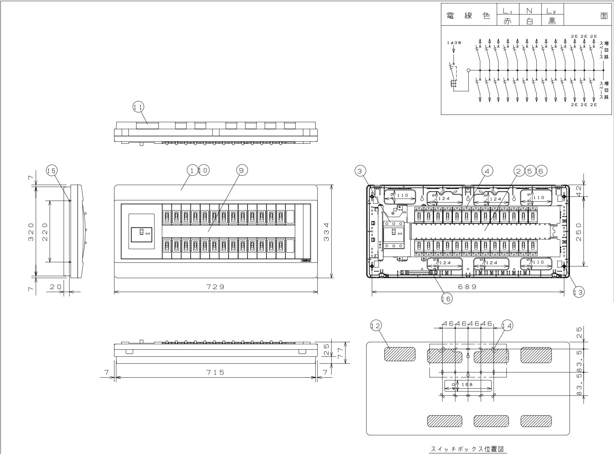
スイッチボックス位置図
