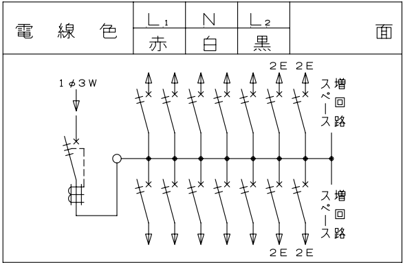
御 納 入 先 様 符号 部 分 品 名 備 考 1 キャビネット スチロール樹脂 2 母線 銅板 100A容量(分岐30A容量) 3 主幹用漏電遮断器 100AF B,C, 5.0kA 30mA 高速形 4 配線用遮断器 30AF B,C, 2.5kA コード短絡保護機能付 5 充電部しゃへい板 ポリプロピレン樹脂 6 200V切替板 銅板 30A 容量 7 8 9 回路銘板 キャビネットカバー表面に貼付 10 100-200V切替説明書 キャビネットカバー裏面に貼付 11 配線用ロックアウト 9 - 30 x 25 12 配 線 孔 13 本体取付ネジ 4 - φ4 x 30 14 スイッチボックス取付穴 5個用スイッチボックス取付可能 15 速結式アース中継端子 M 5 x 2 , 速結端子10P 16 17 18 19
