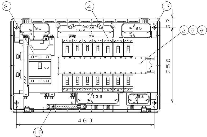
御 納 入 先 様 符号 部 分 品 名 備 考 1 キャビネット スチロール樹脂 2 母線 銅板 100A容量(分岐30A容量) 3 主幹用漏電遮断器 100AF B,C, 5.0kA 30mA 高速形 4 配線用遮断器 30AF B,C, 2.5kA コード短絡保護機能付 5 充電部しゃへい板 ポリプロピレン樹脂 6 200V切替板 銅板 30A 容量 7 8 9 回路銘板 キャビネットカバー表面に貼付 10 100-200V切替説明書 キャビネットカバー裏面に貼付 11 配線用ロックアウト 9 - 30 x 25 12 配 線 孔 13 本体取付ネジ 4 - φ4 x 30 14 スイッチボックス取付穴 5個用スイッチボックス取付可能 15 速結式アース中継端子 M 5 x 2 , 速結端子10P 16 17 18 19
