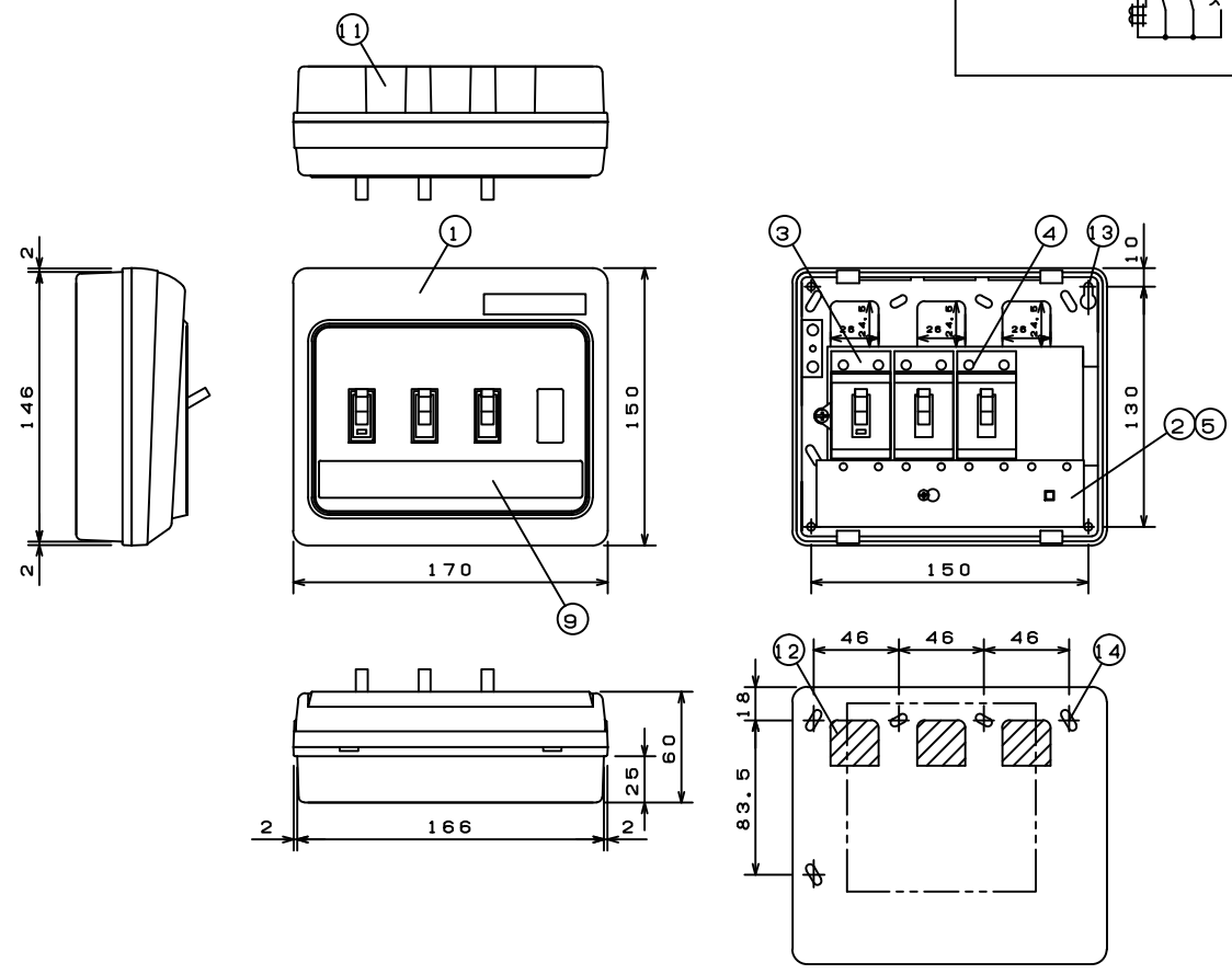
スイッチボックス位置図
