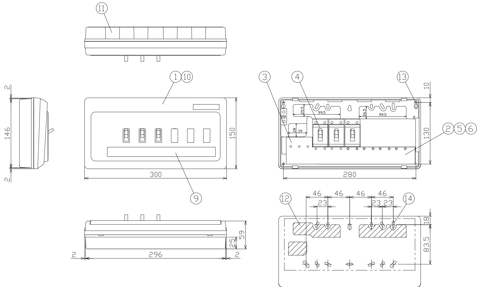
スイッチボックス位置図
