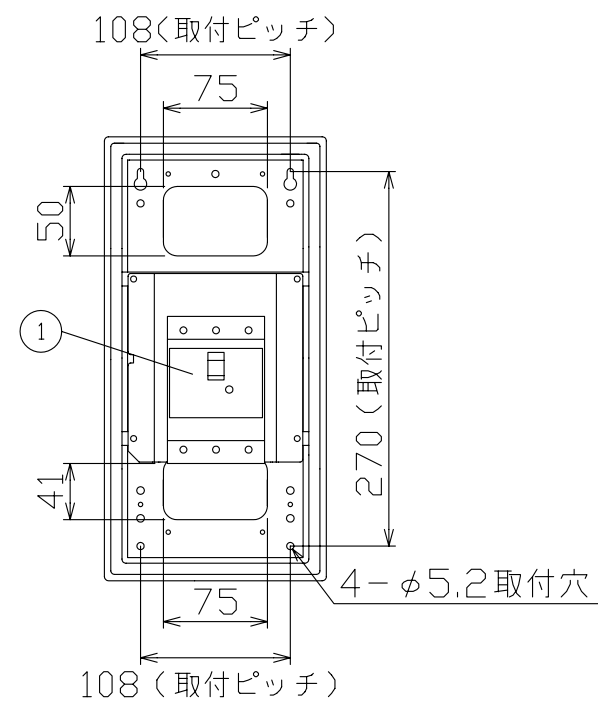
配線孔寸法図<////部開口>
