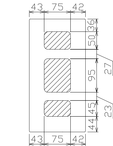
配線孔寸法図<////部開口>
