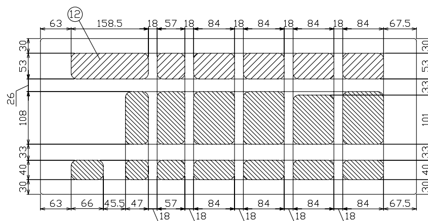
配線孔寸法図
