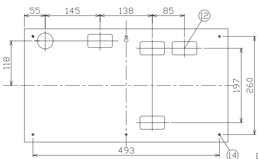
ケース底面ロックアウト図
