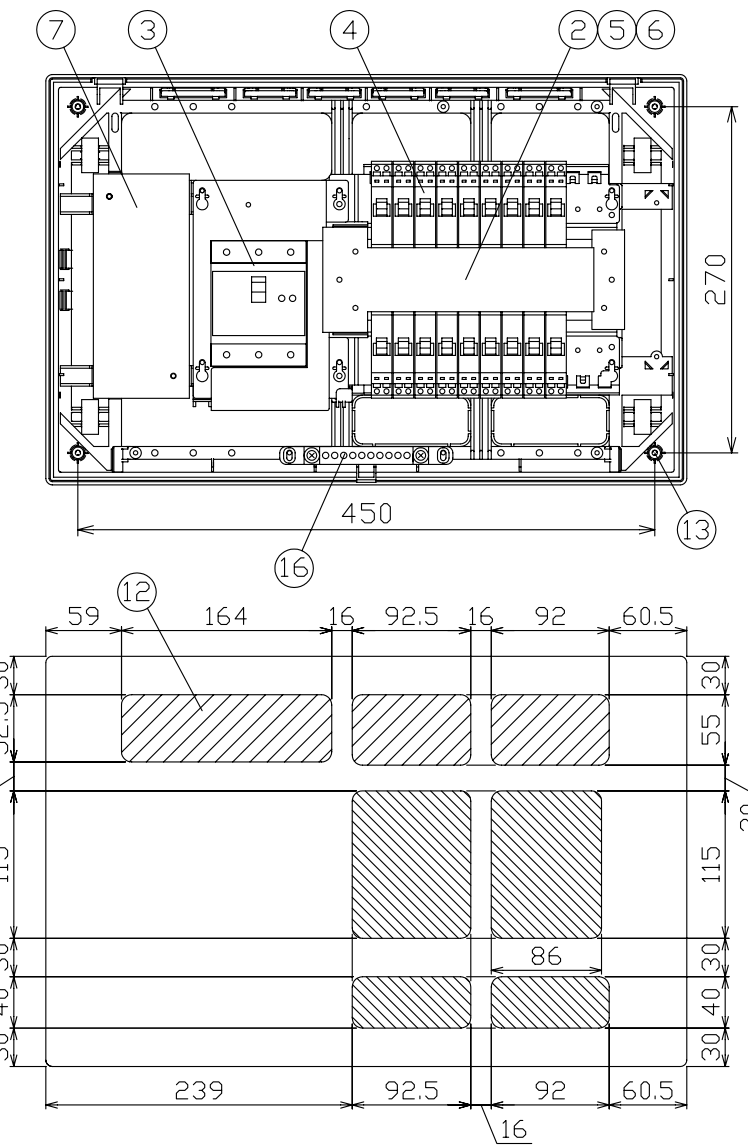
配線孔寸法図
