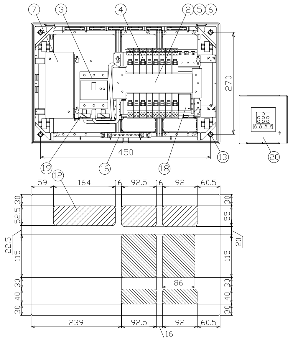
配線孔寸法図
