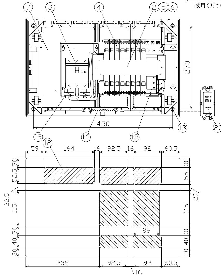
配線孔寸法図
