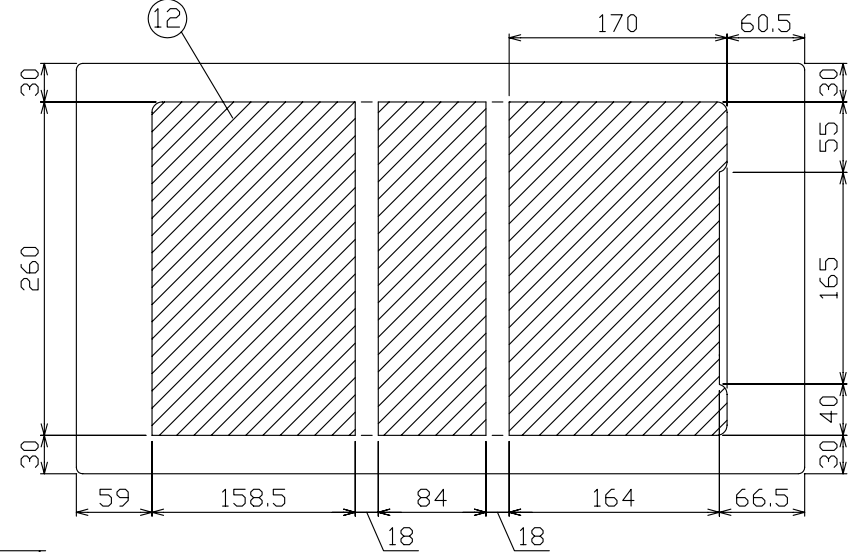
配線孔寸法図
