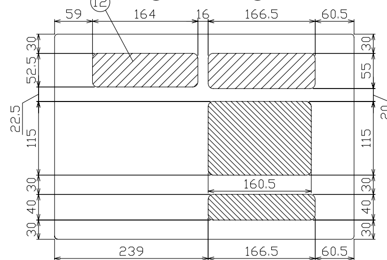
配線孔寸法図
