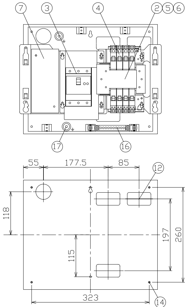
ケース底面ノックアウト図
