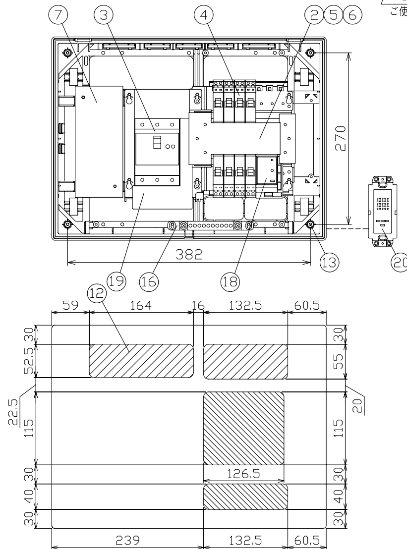
配線孔寸法図
