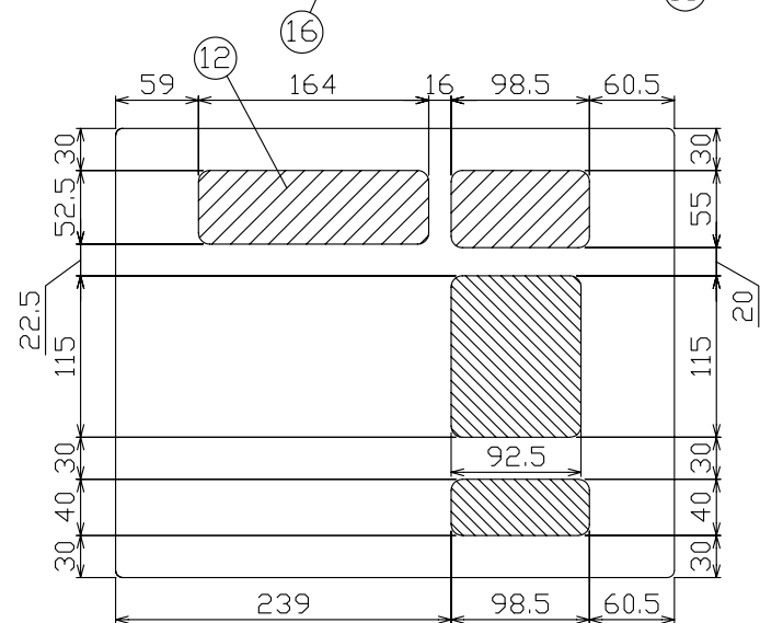
配線孔寸法図
