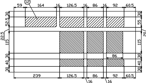
配線孔寸法図
