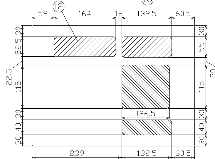
配線孔寸法図
