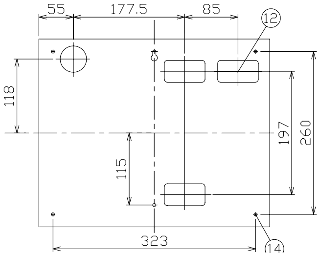
ケース底面ノックアウト図
