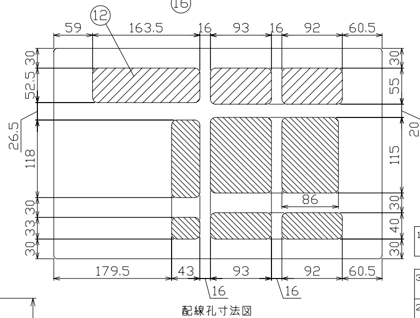
配線孔寸法図
