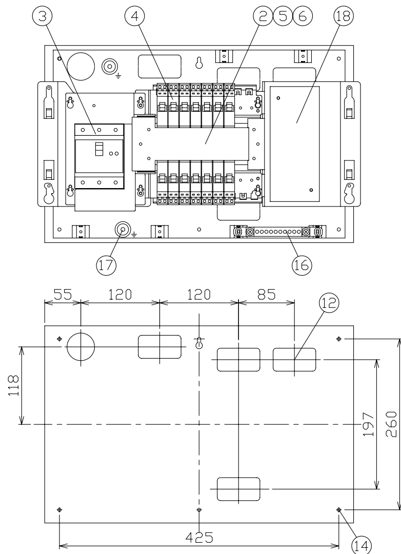
ケース底面ノックアウト図
