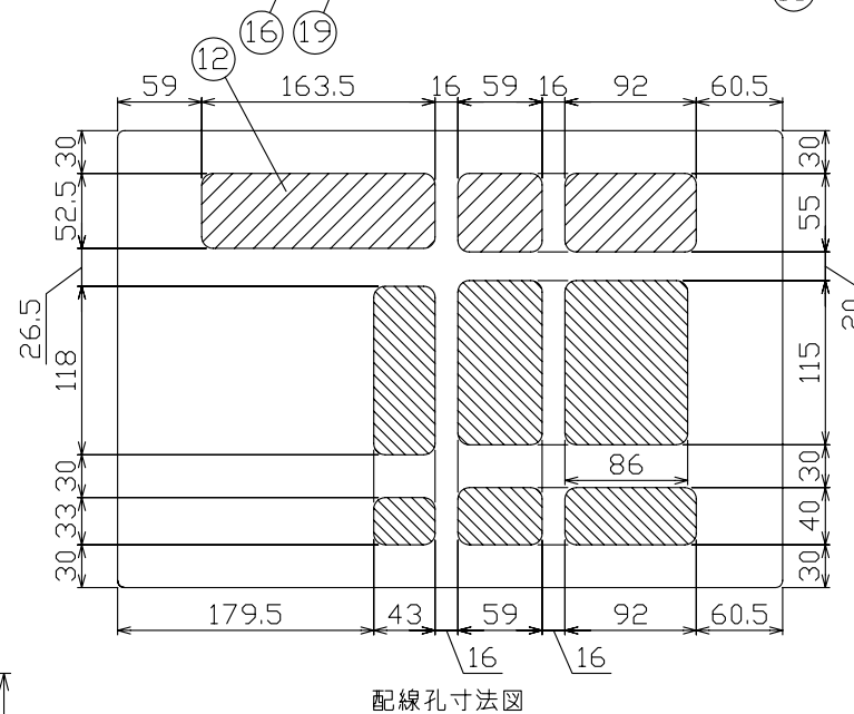
配線孔寸法図
