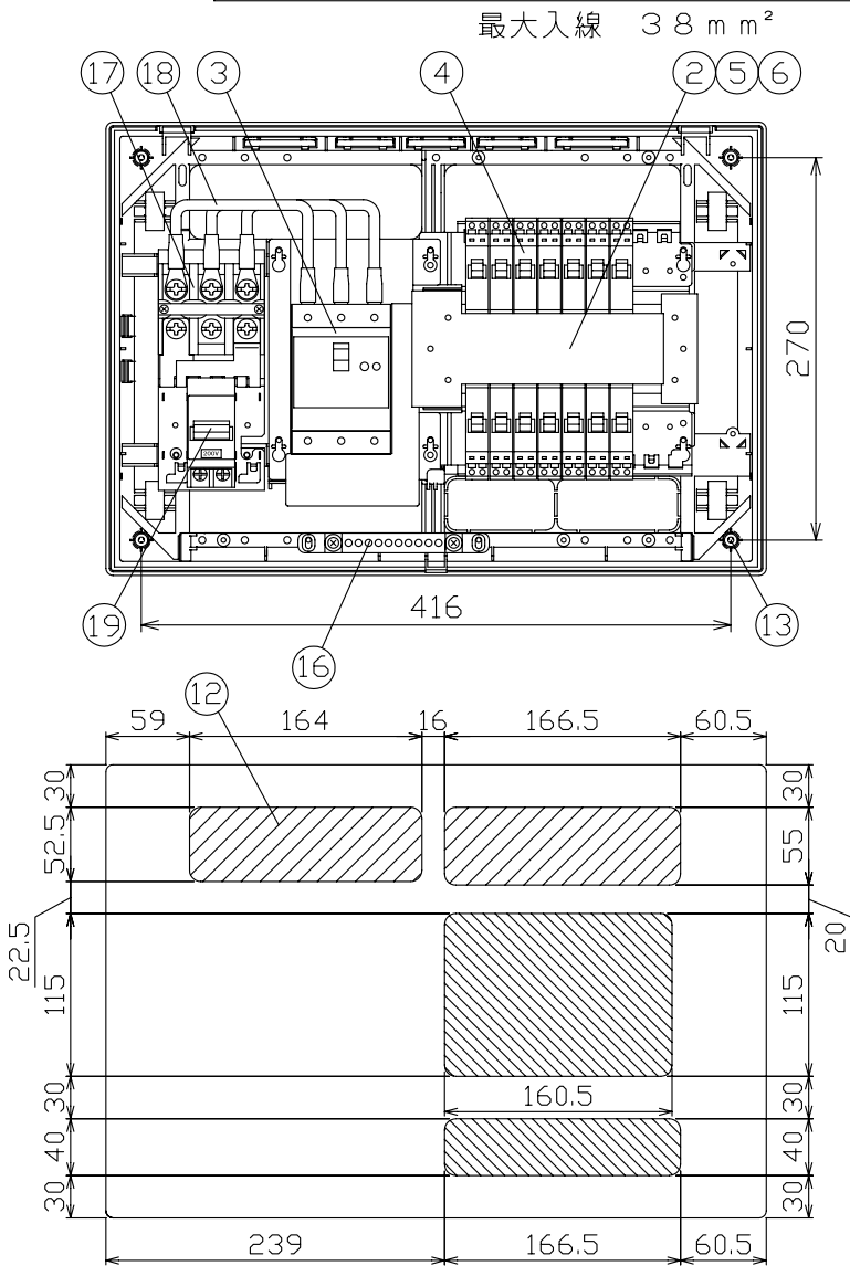
配線孔寸法図
