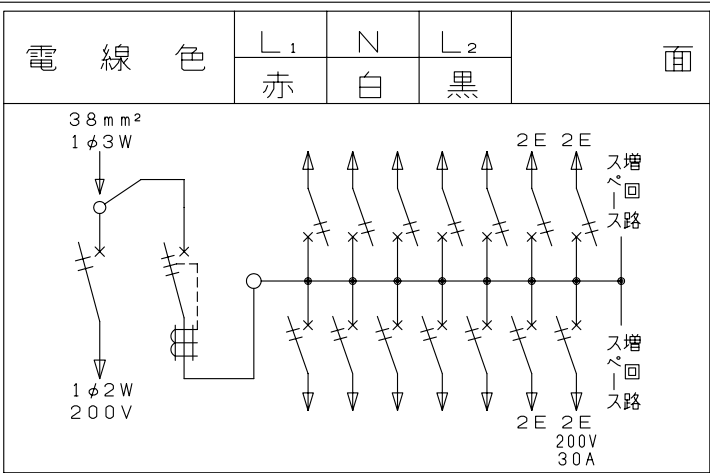
御 納 入 先 様 符号 部 分 品 名 備 考 1 キャビネット スチロール樹脂 UL-94 V-2 2 母線 銅板 60A容量(分岐30A容量) 3 主幹用漏電遮断器 60AF B,C, 5.0kA 30mA高速形 4 配線用遮断器 30AF B,C, 2.5kA コード短絡保護機能付 5 充電部しゃへい板 ポリプロピレン樹脂 6 200V切替板 銅板 30A 容量 7 8 9 回路銘板 キャビネットカバー表面に貼付 10 100-200V切替説明書 キャビネットカバー裏面に貼付 11 配 線 孔 ノックアウト式 12 配 線 孔 \\\\\\\\ 部開口, \\\\\\\生 部ノックアウト式 13 本体取付ネジ 4 - φ4.5 x 30 14 15 半埋込取付用サイドノック 4 - φ5 16 速結式アース中継端子 M 5 x 2 , 速結端子10P 17 端 子 台 日東工業(株)製 TBF-103 端子ネジM8 18 電線(端子台～主幹) 600V EM-IE 電線 14mm 2 19 電気温水器用配線用遮断器 30AF B,C, 2.5kA コード短絡保護機能付 20 温水器用シール キャビネットカバー表面に貼付
